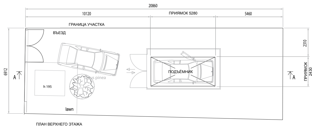
ПЛАН ВЕРХНЕГО ЭТАЖА
