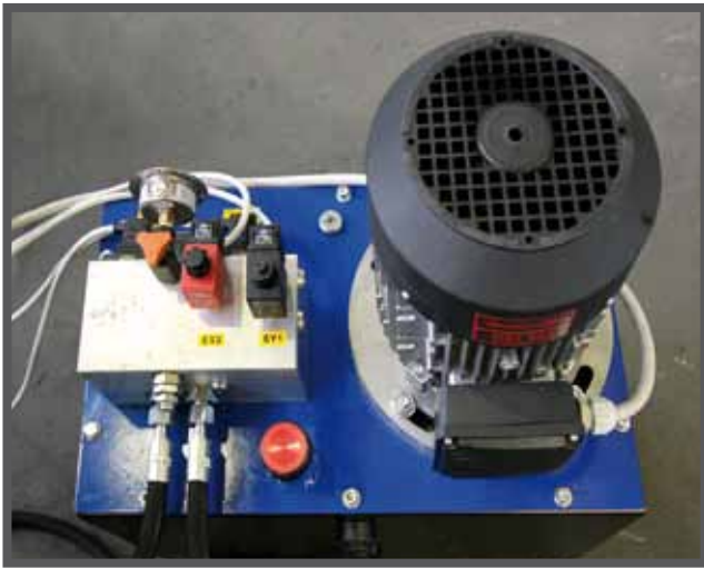
На общем виде электрогидравлического блока хорошо видны его компактные размеры: (монтаж не требует много места).
