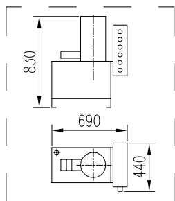
ГИДРОСТАНЦИЯ
