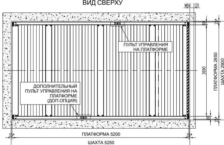
ВИД СВЕРХУ
