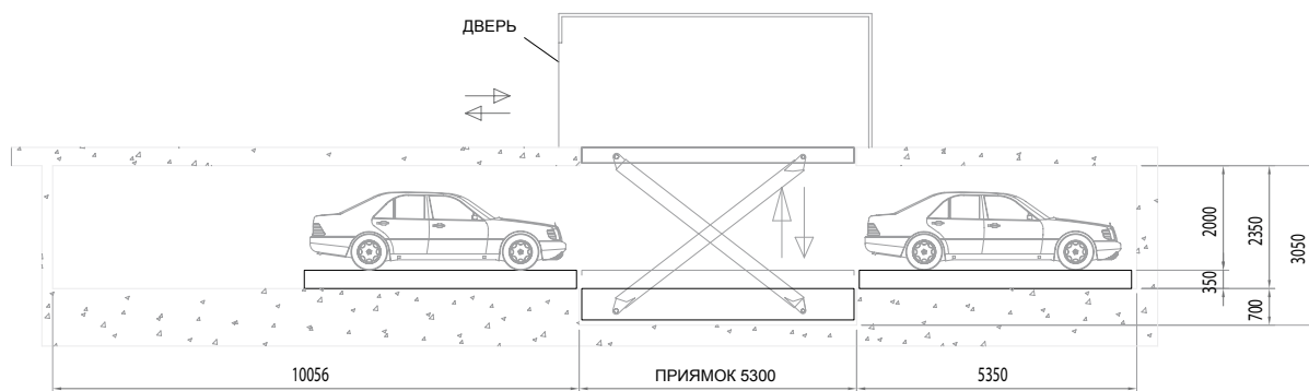
СБОКУ А-А
