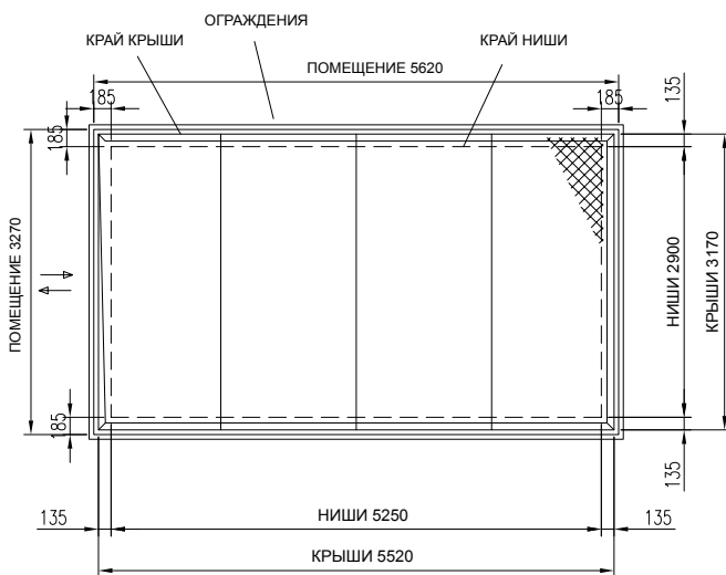
КРЫША ВИД С ВЕРХУ
