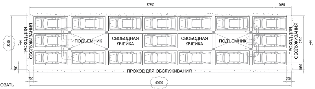
ПЛАН ПАРКОВКИ
