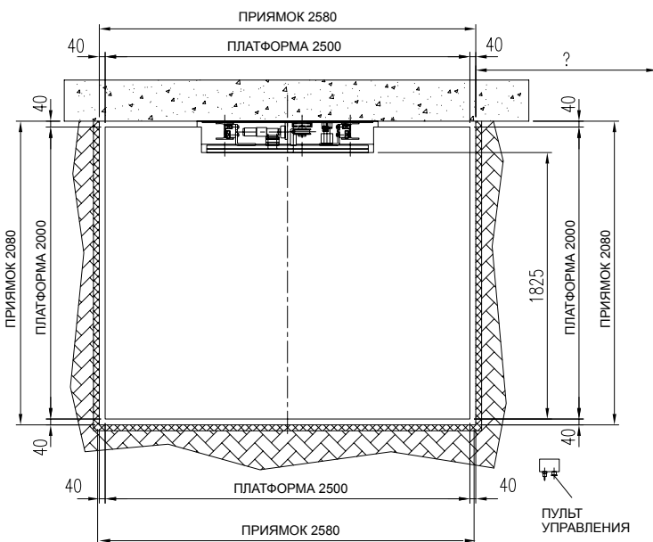
ВИД СВЕРХУ
