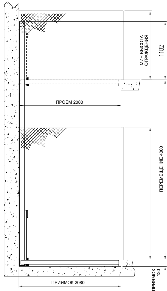
ВИД СБОКУ
