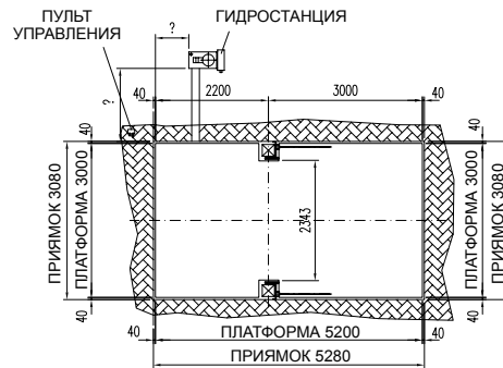
ПЛАН ВЕРХНЕГО ЭТАЖА
