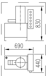
ГИДРОСТАНЦИЯ
