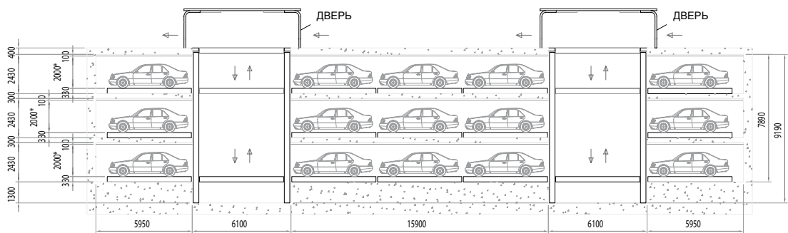
РАЗРЕЗ А-А
