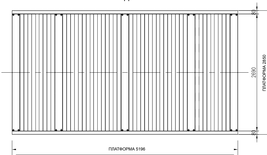
ВИД СВЕРХУ
